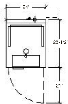
BM23 Top
