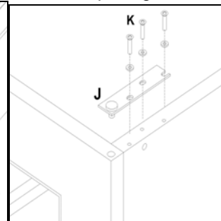
Top Hinge
