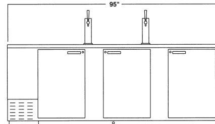
DD94 Front
