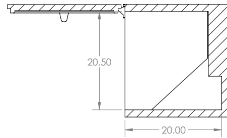
SECTION A-A SCALE 1 : 12
